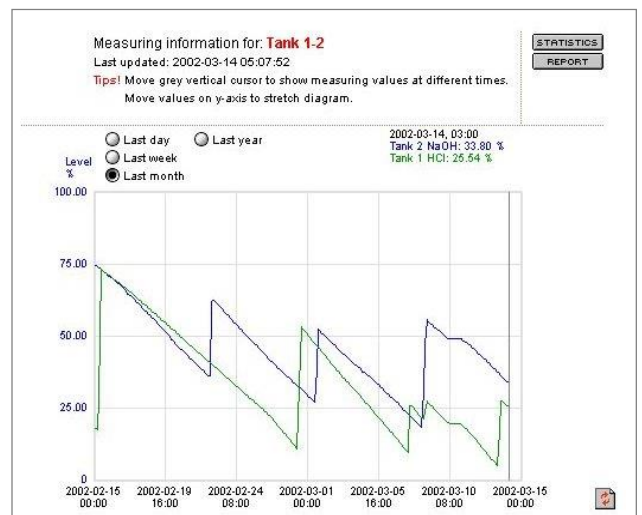
Mätning av nivå i tankar.
